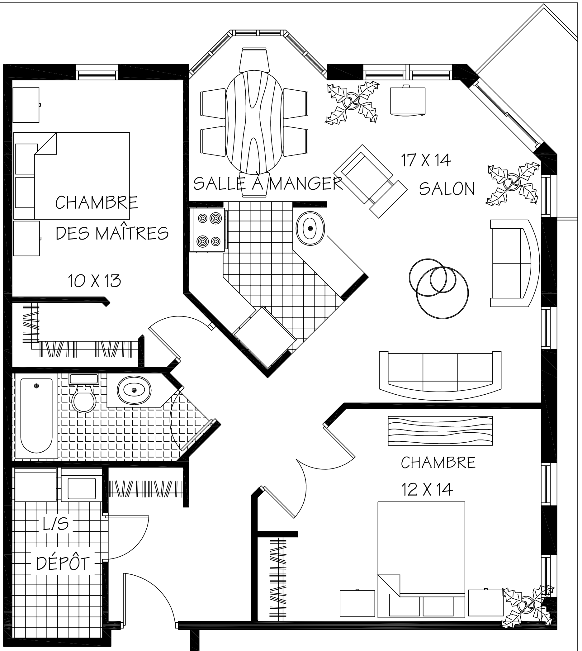
MODÈLE DE TYPE 2 CHAMBRES (16)
